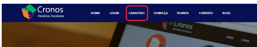
Figura 2 - Menu superior
