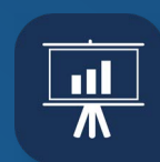
Power BI
