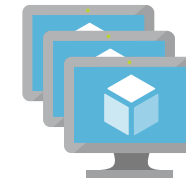
仮想マシン
