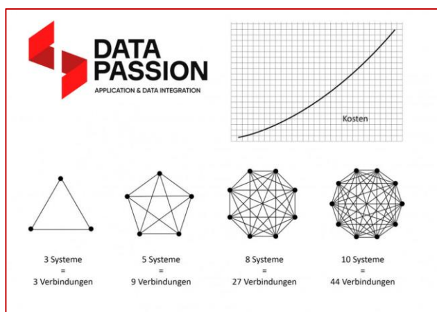
Punkt-zu-Punkt- vs. ESB-Integration
