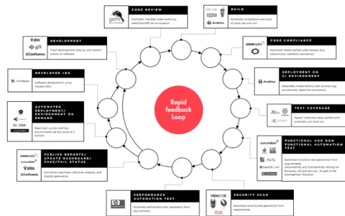
DevSecOps
